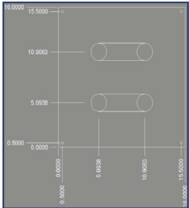
PP-158- 4U
