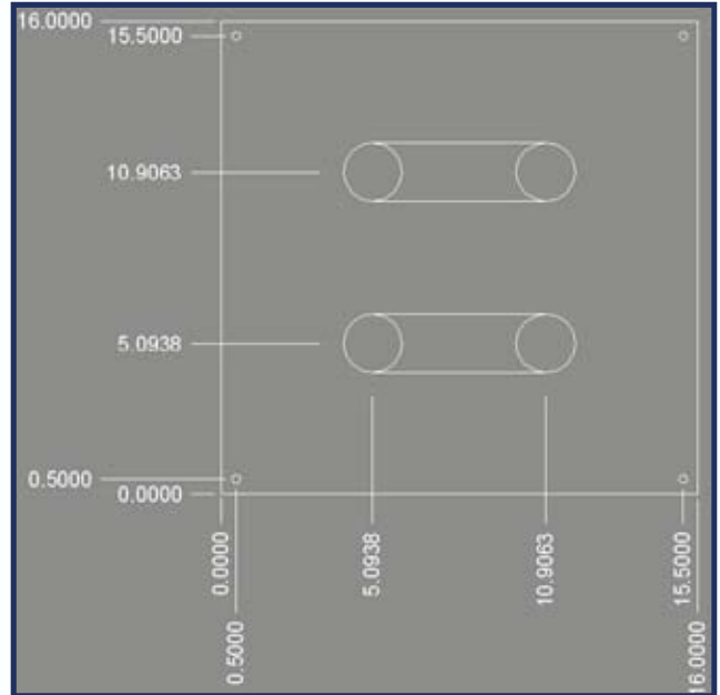
PP-318- 4U
