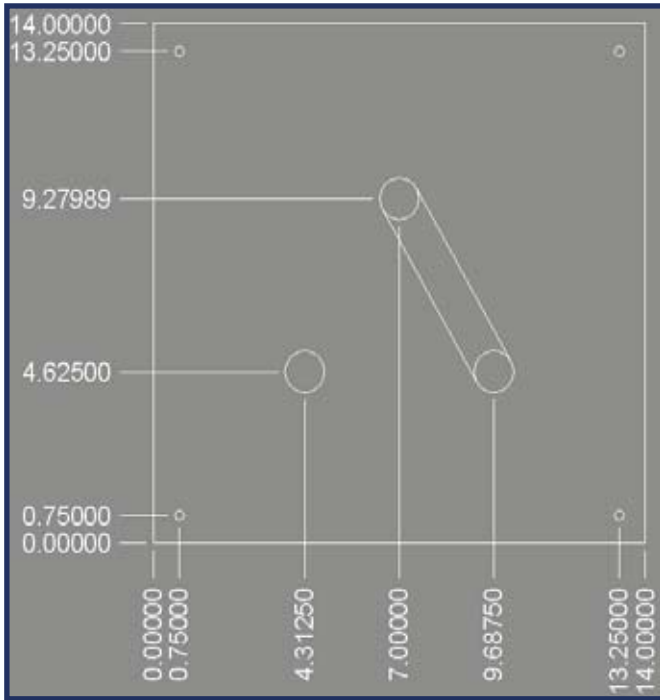
PP-78- 3U
