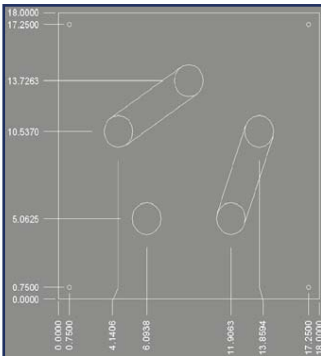
PP-158- 5U
